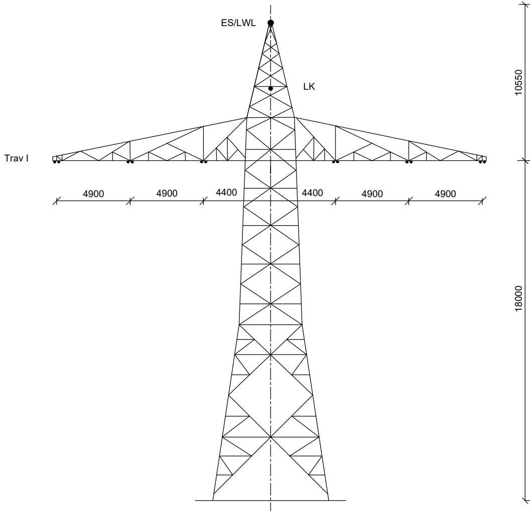
WAVE 100-18 B58: Mast Nr. 2neu
