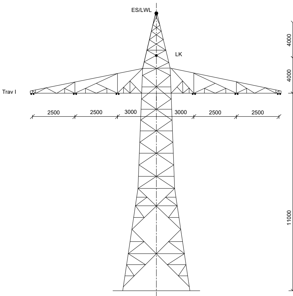
WE/WAdiff/120-11.00 B57: Mast Nr. 1a
