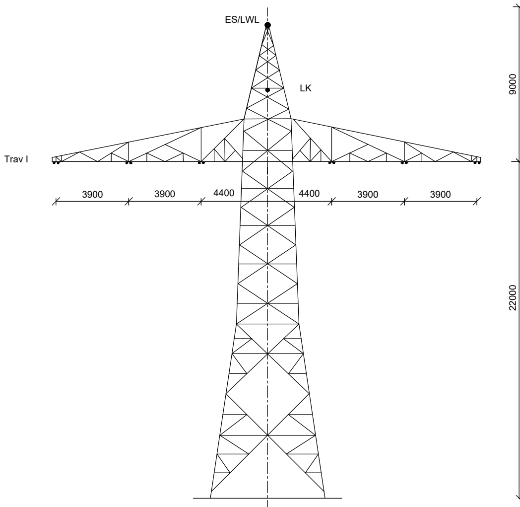
WA140-22.00 B57: Mast Nr. 21neu
