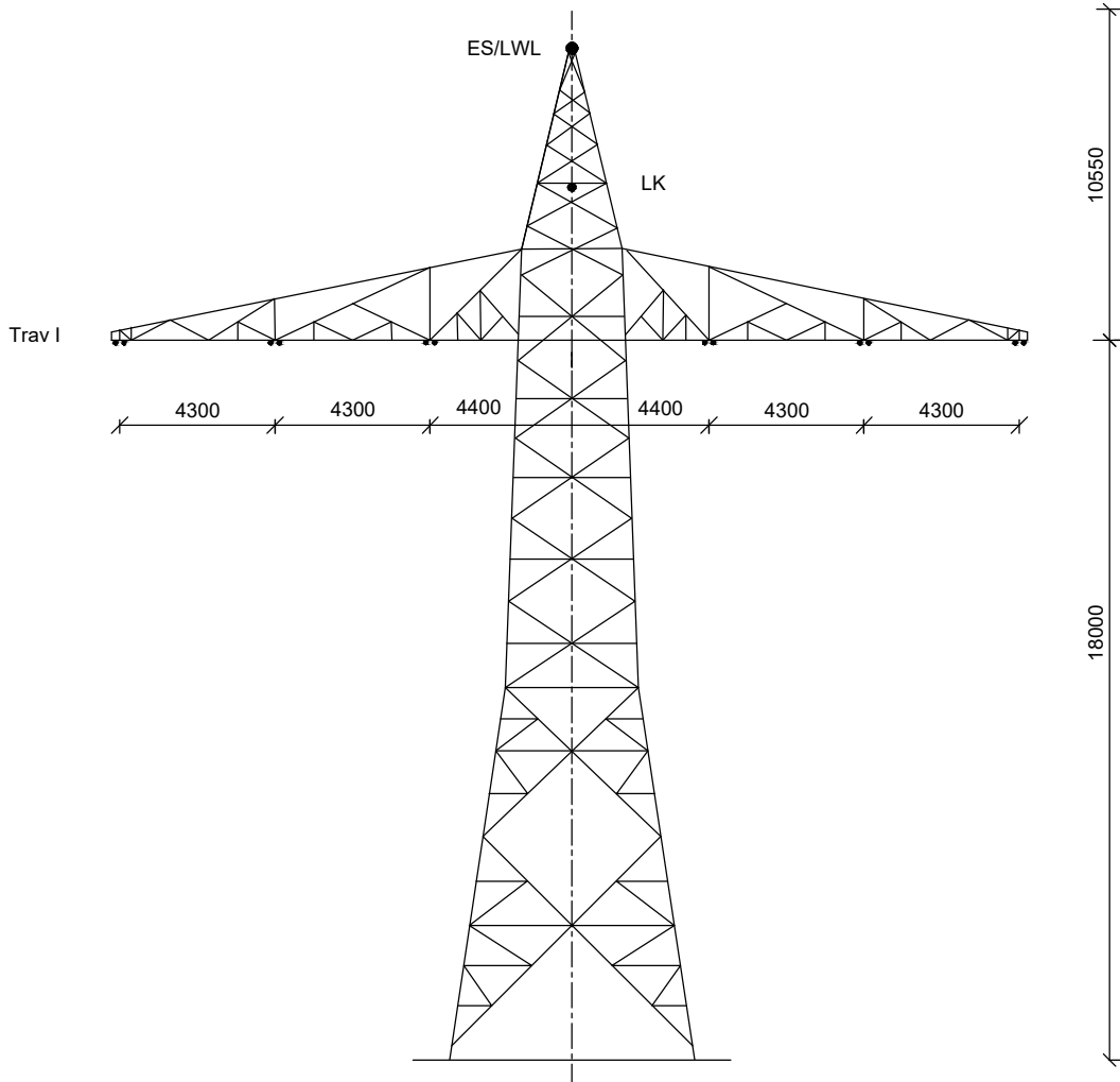
WA120-18 B58: Mast Nr. 3neu
