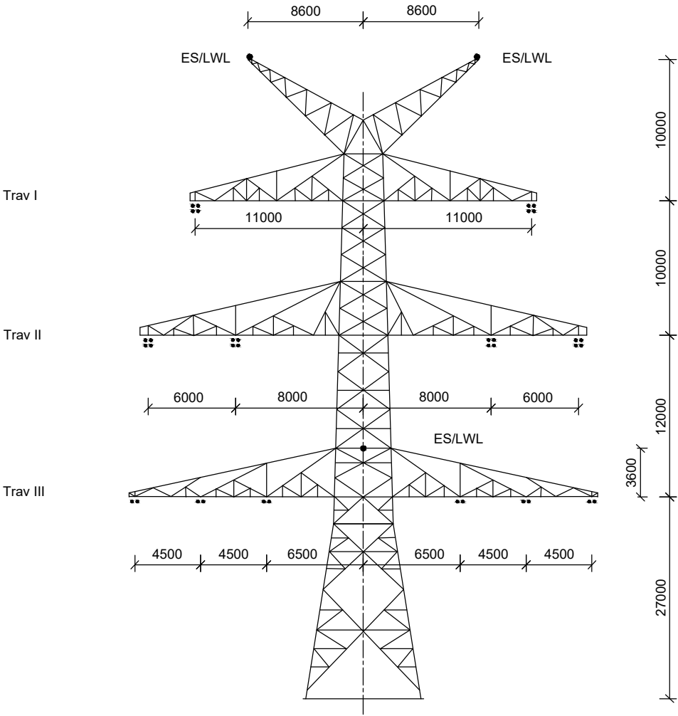
WA160-27.00 B175: Mast Nr. 2A, 3A
