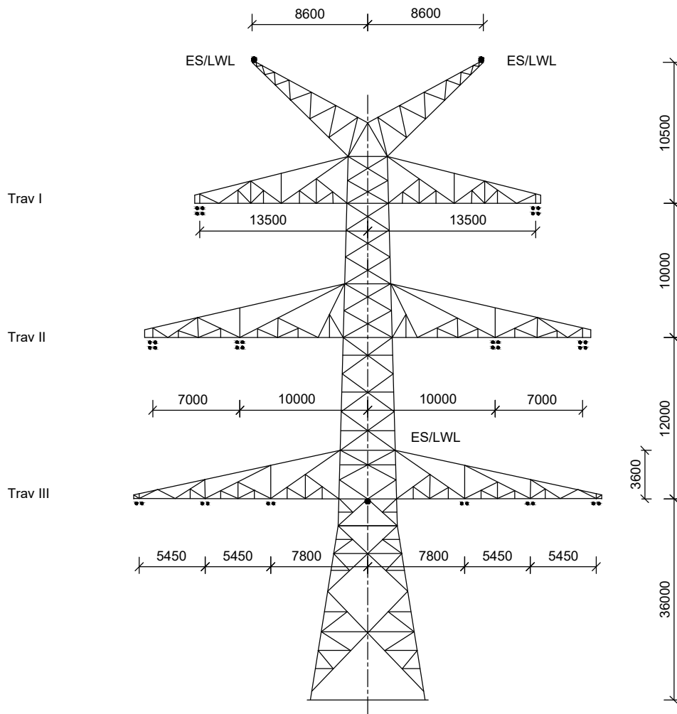
WA120-36.00 B175: Mast Nr. 6A
